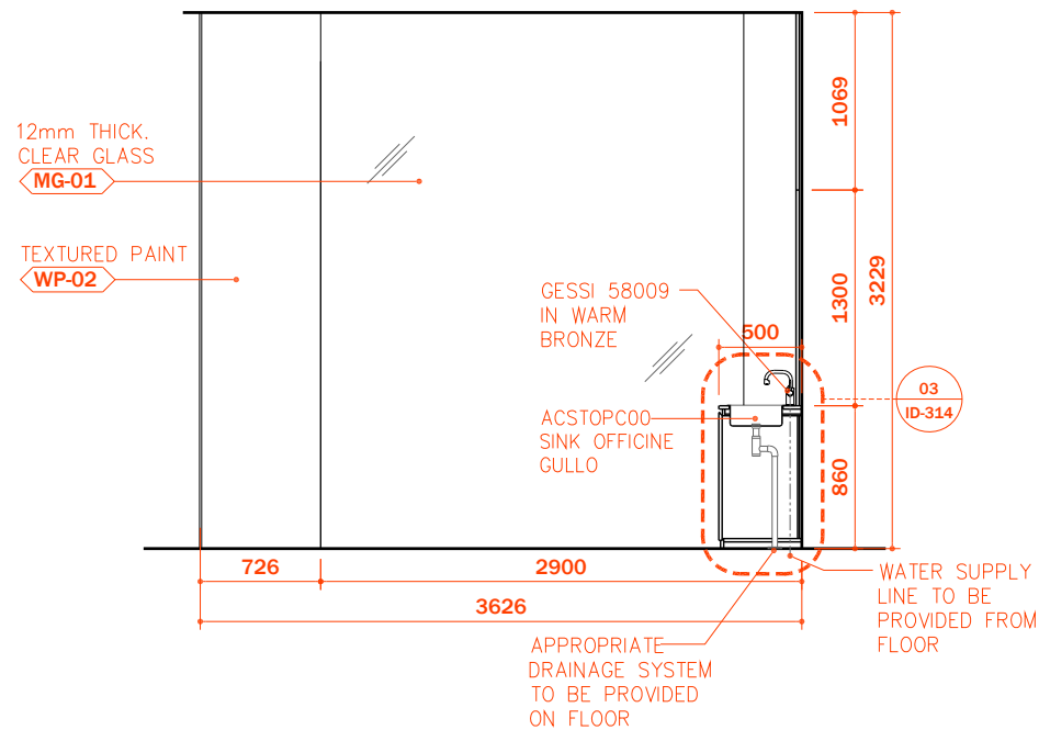
04 ELEVATION
