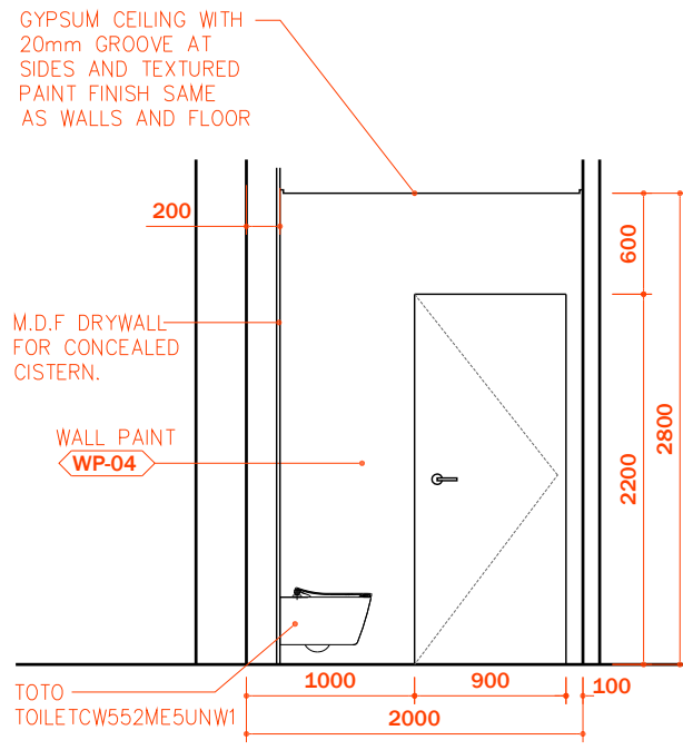
06 ELEVATION
