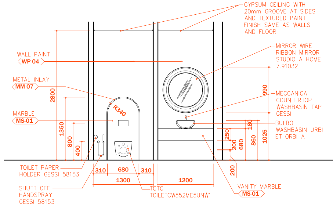
01 ELEVATION
