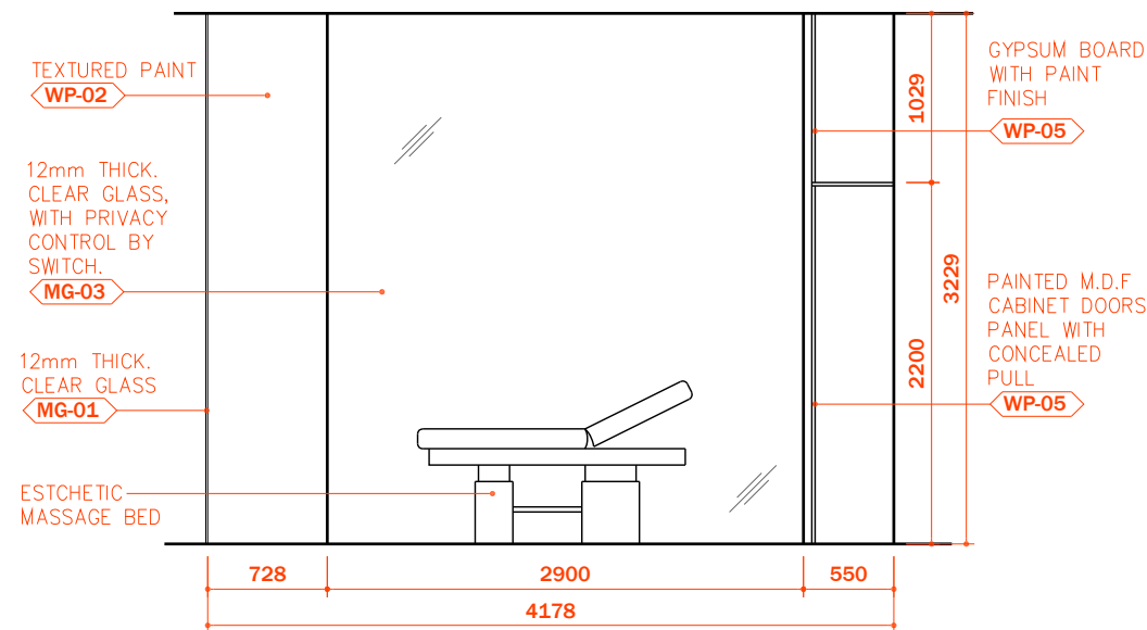
04 ELEVATION
