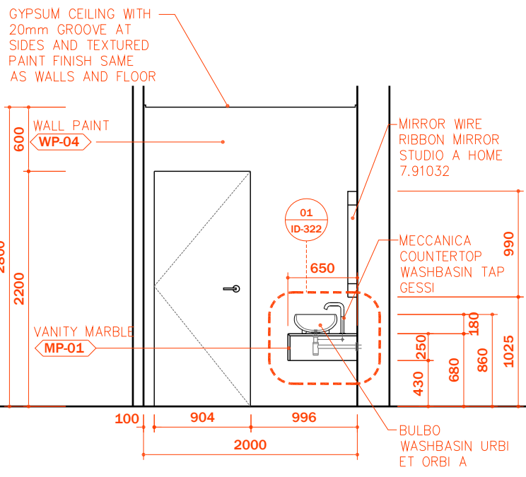
04 ELEVATION
