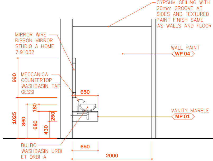
02 ELEVATION
