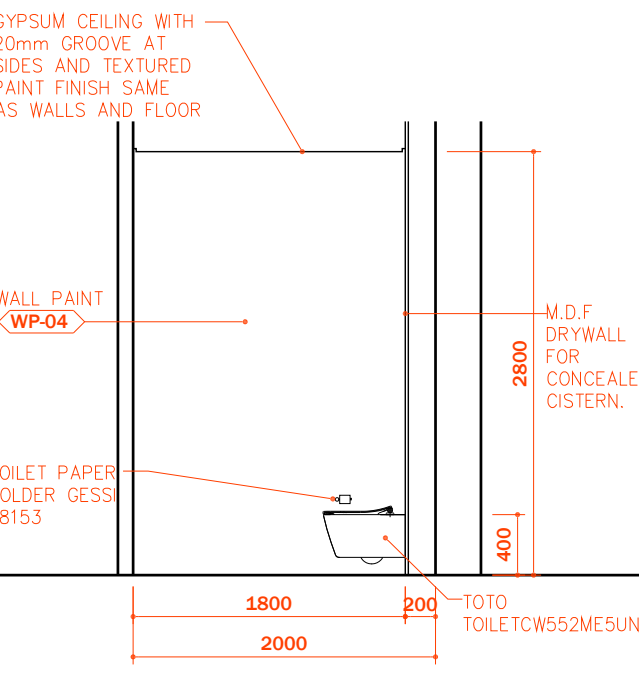
05 ELEVATION
