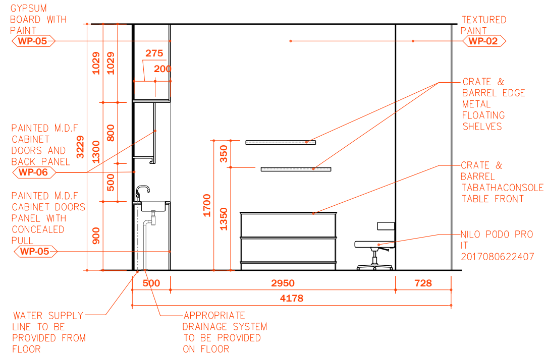
02 ELEVATION
