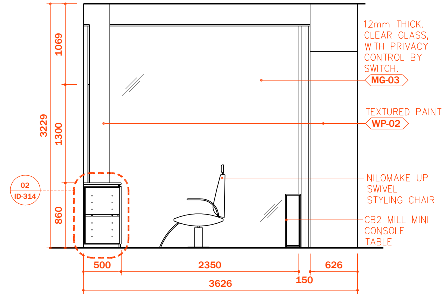
02 ELEVATION
