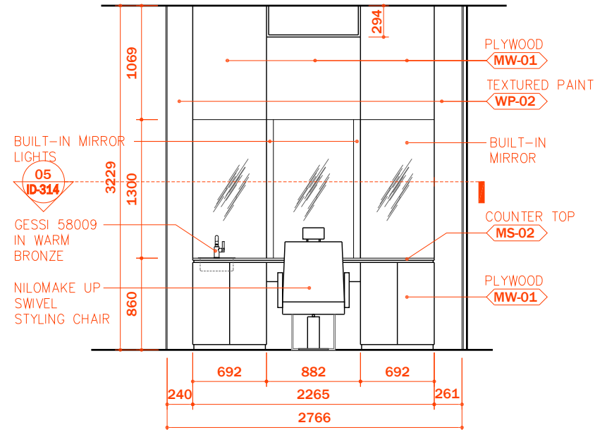
01 ELEVATION
