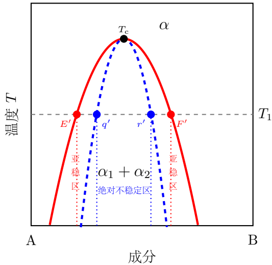
溶混间隙相图
