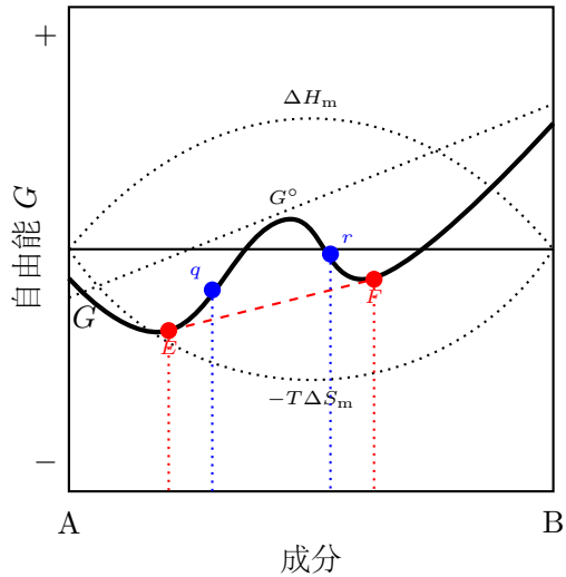
T_1 下的自由能-成分曲线 ( \Omega > 0 )
