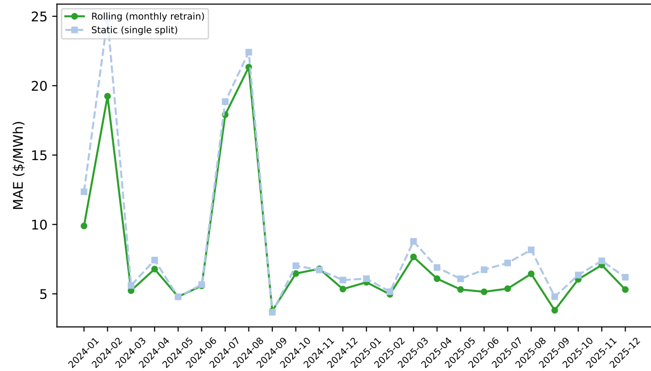
ERCOT: XGBoost
