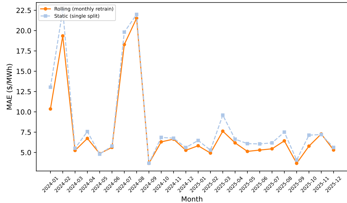
ERCOT: XGBoost
