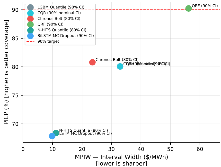
ERCOT — PICP vs. MPIW
