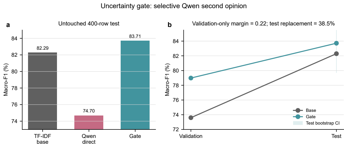
图 7 选择性 Qwen 二次意见。a，固定 400 条测试集的 TF-IDF 基线、Qwen 直接分类和门控结果；b，验证集选择的区间迁移到测试集后的变化，浅色带为测试集配对 bootstrap 95% CI。门控提升为探索性点估计，CI 跨过 0。
