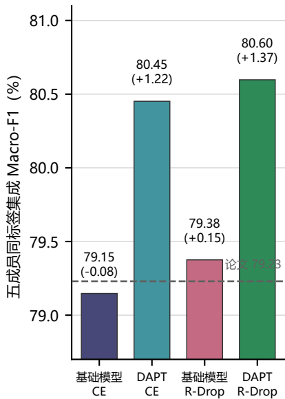
b 2×2 消融：主要增益来自 DAPT
