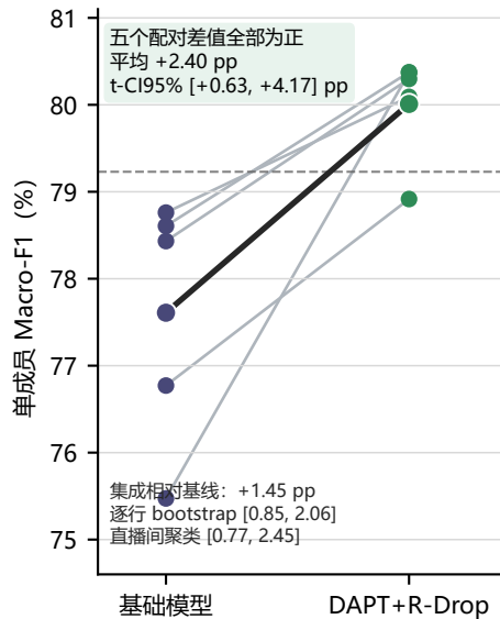
c 同种子配对：提升不是单个幸运初始化
