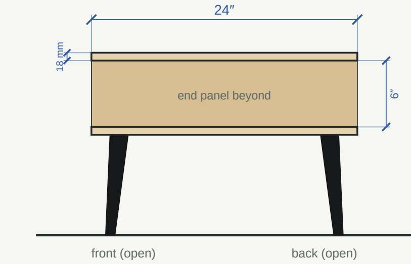
5 Section A-A
