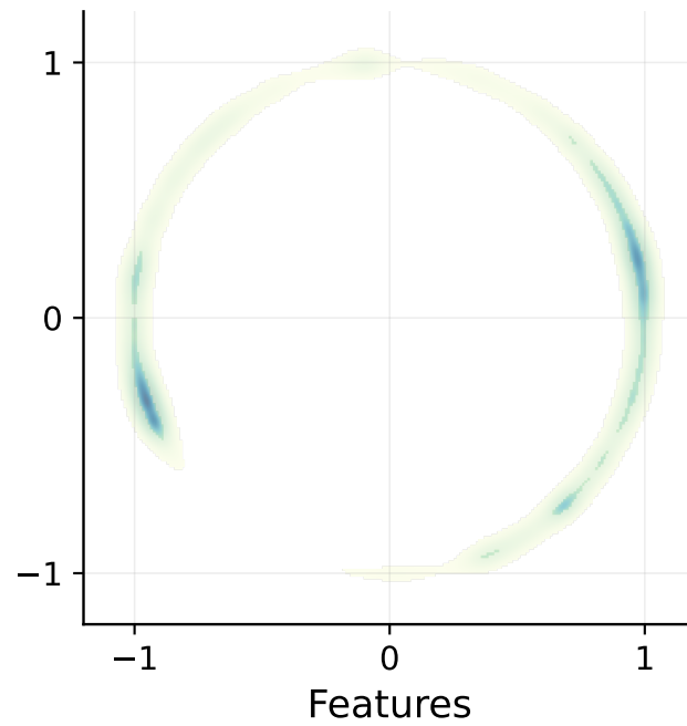
AlphaEarth
