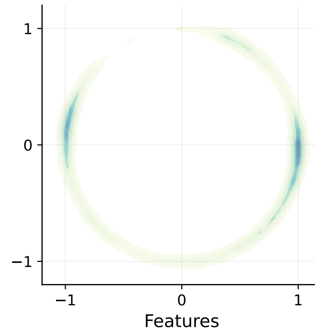
TESSERA
