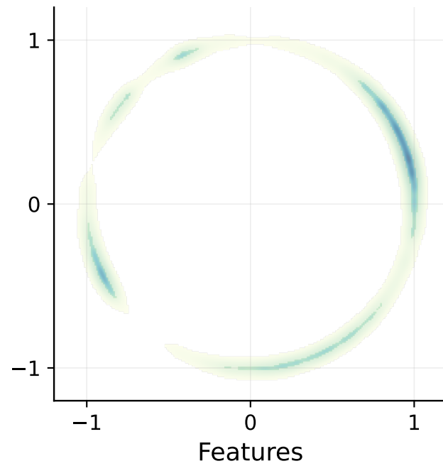
Basin2Vec
