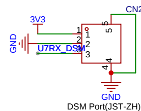
DSM Port(JST-ZH)
