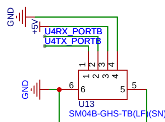
PortB(JST-GH) Default FUNC : UART4 Reuse FUNC : 2*Timer_Chx
