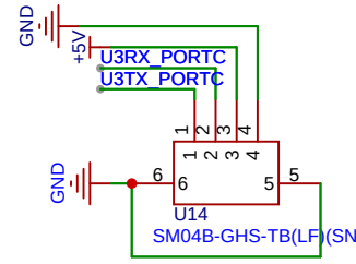
PortC(JST-GH) Default FUNC : UART3
