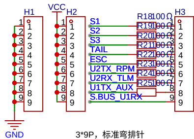
3*9P, 标准弯排针
