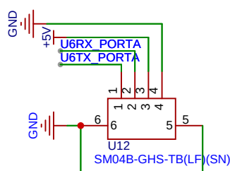
PortA(JST-GH) Default FUNC : UART6 Reuse FUNC : 2*RPM or 2*ADC_Chx
