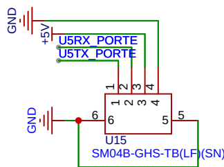
PortE(JST-GH) Default FUNC : UART5 如果板载接收机, 该接口直接接到内部接收机, 常用于GPS+罗盘 去掉该接口
