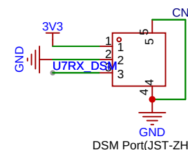
DSM Port(JST-ZH)
