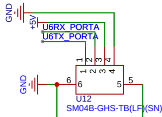
PortA(JST-GH) Default FUNC : UART6 Reuse FUNC : 2*RPM or 2*ADC_Chx
