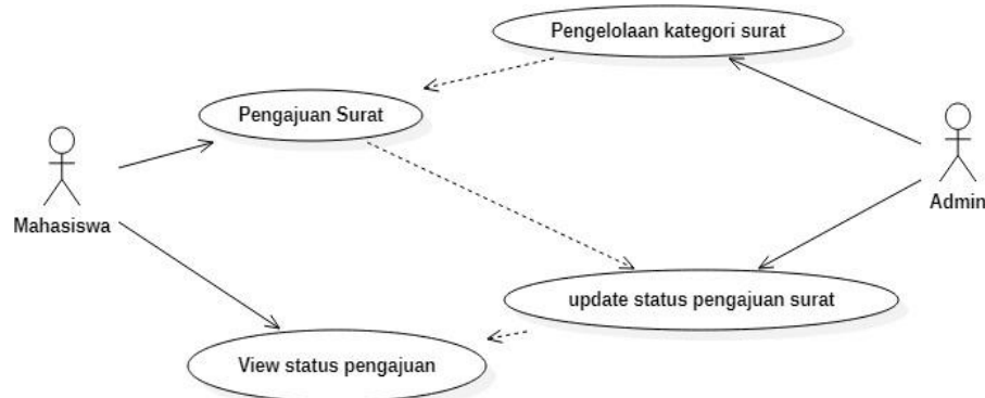
Gambar 1. Usecase sistem pengelolaan administrasi surat
