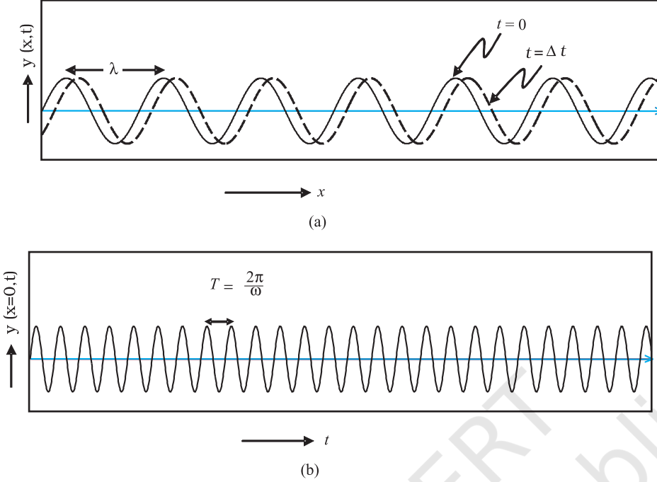
चित्र 10.17 (a) वक्र किसी डोरी का क्रमशः t = 0 तथा t = \Delta t पर विस्थापन निरूपित करते हैं, जब एक ज्यावक्र्रीय तरंग +x दिशा में संचरित होती है। (b) वक्र विस्थापन x = 0 के समय-विचरण को निरूपित करता है, जबकि एक ज्यावक्र्रीय तरंग +x दिशा में संचरित हो रही है। x = \Delta x पर विस्थापन का समय-विचरण थोड़ा-सा दाईं ओर विस्थापित हो जाएगा।
