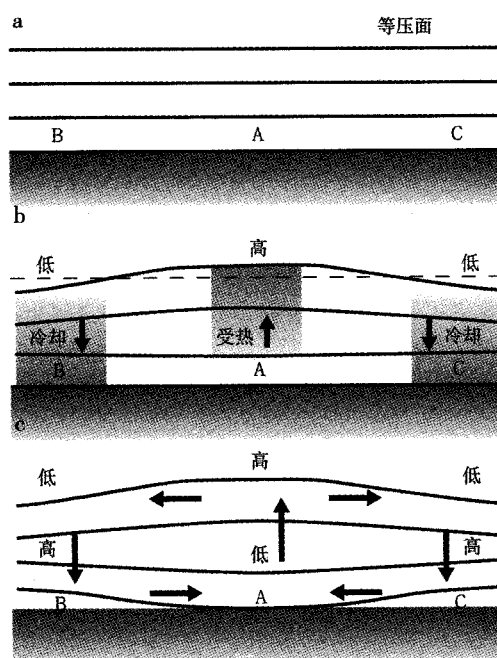
图 2.3 热力环流的形成
