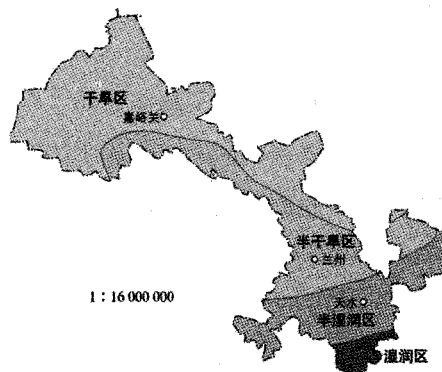
图 1-1-3 甘肃省干湿区的划分
