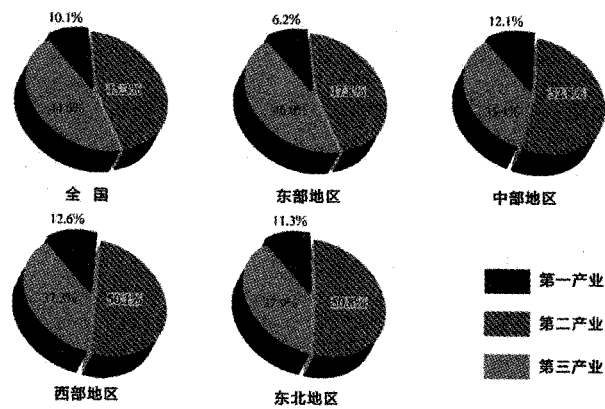
图 1-13 2012 年我国四大地区产业结构比较
