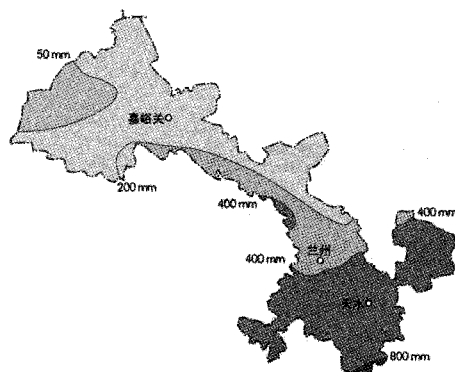
图 1-1-2 甘肃省年降水量分布
