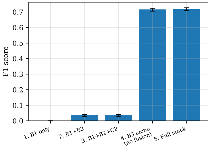
Layer Ablation -- F1 with 95% Bootstrap CI (n=10,000)
