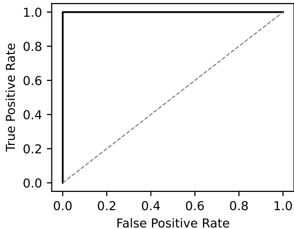
ROC (AUC=1.0000)
