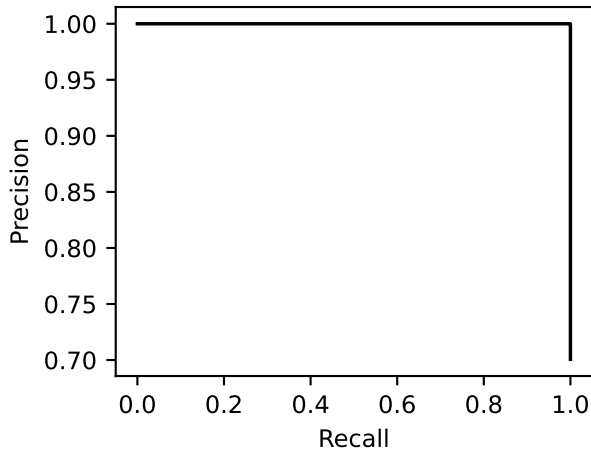
PR (AUC=1.0000)
