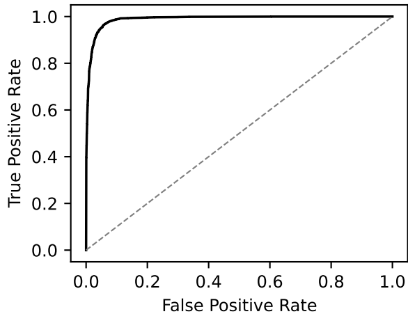
ROC (AUC=0.9892)
