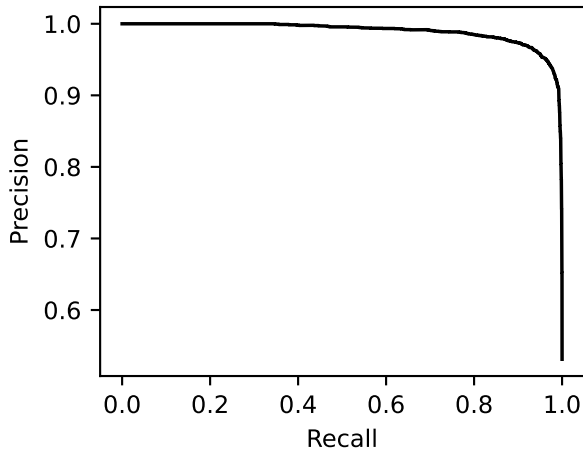
PR (AUC=0.9896)
