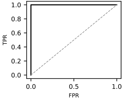
ROC (AUC=1.000)
