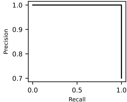
PR (AUC=1.0000)
