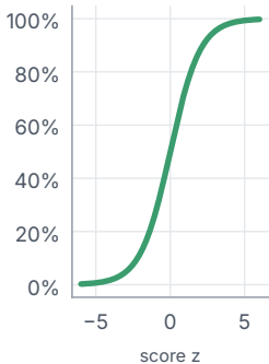
noul \rightarrow P(yes)
