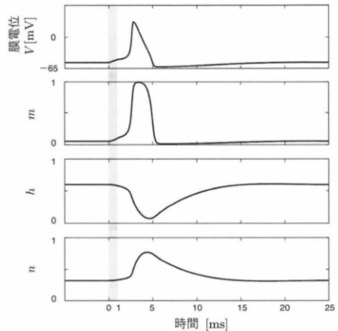
Hodgkin-Huxley モデル膜電位応答[3]
