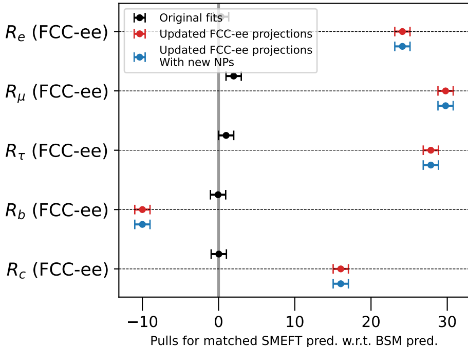
IDM (BP 2), FCC-ee 240 + FCC-ee 365
