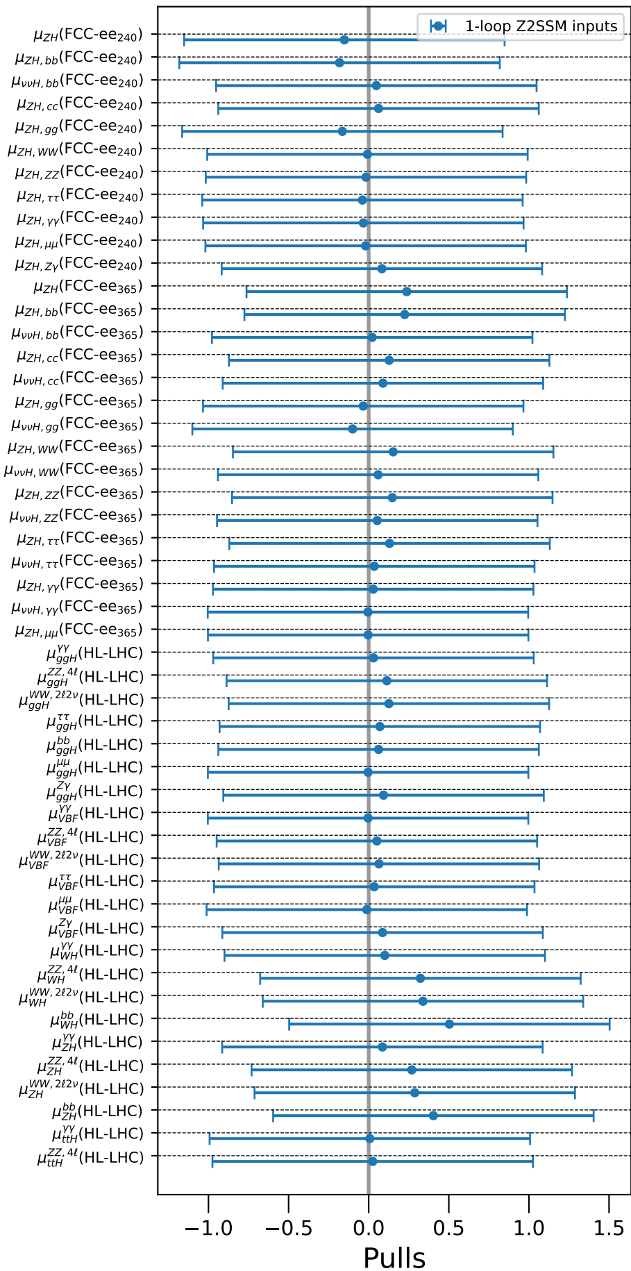
Z2SSM (BP 1), FCC-ee 240 + FCC-ee 365
