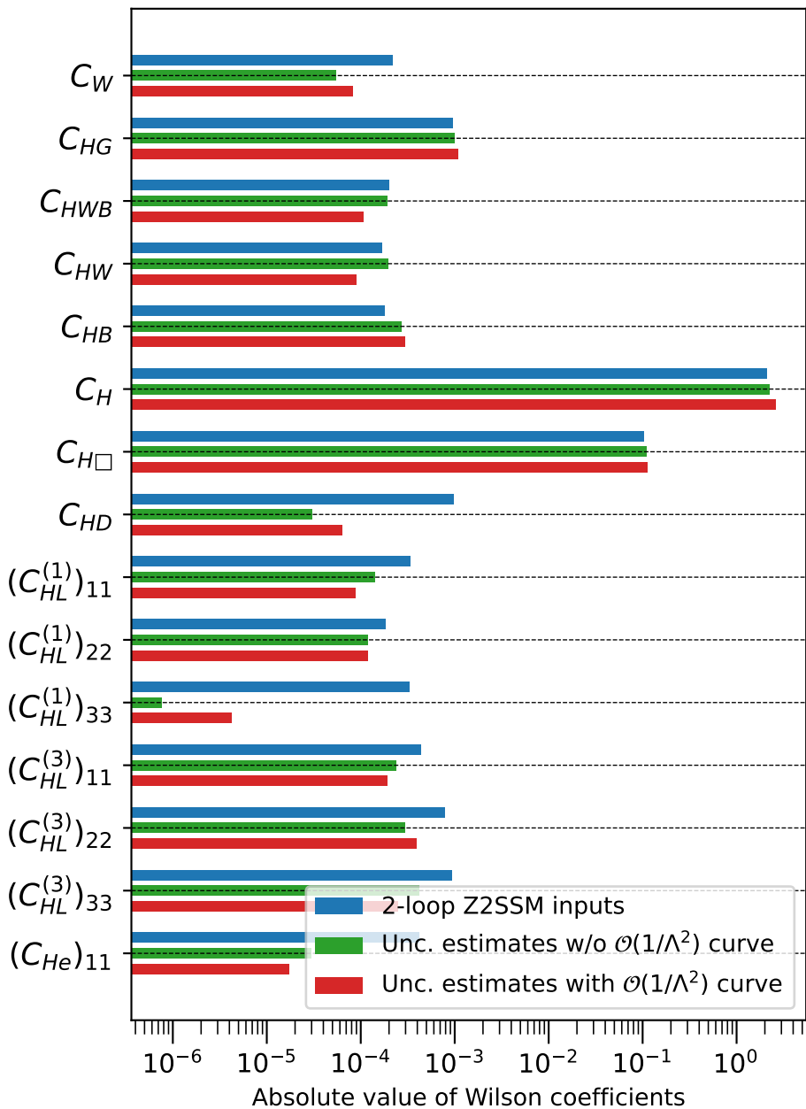
Z2SSM (BP 1), FCC-ee 240 + FCC-ee 365
