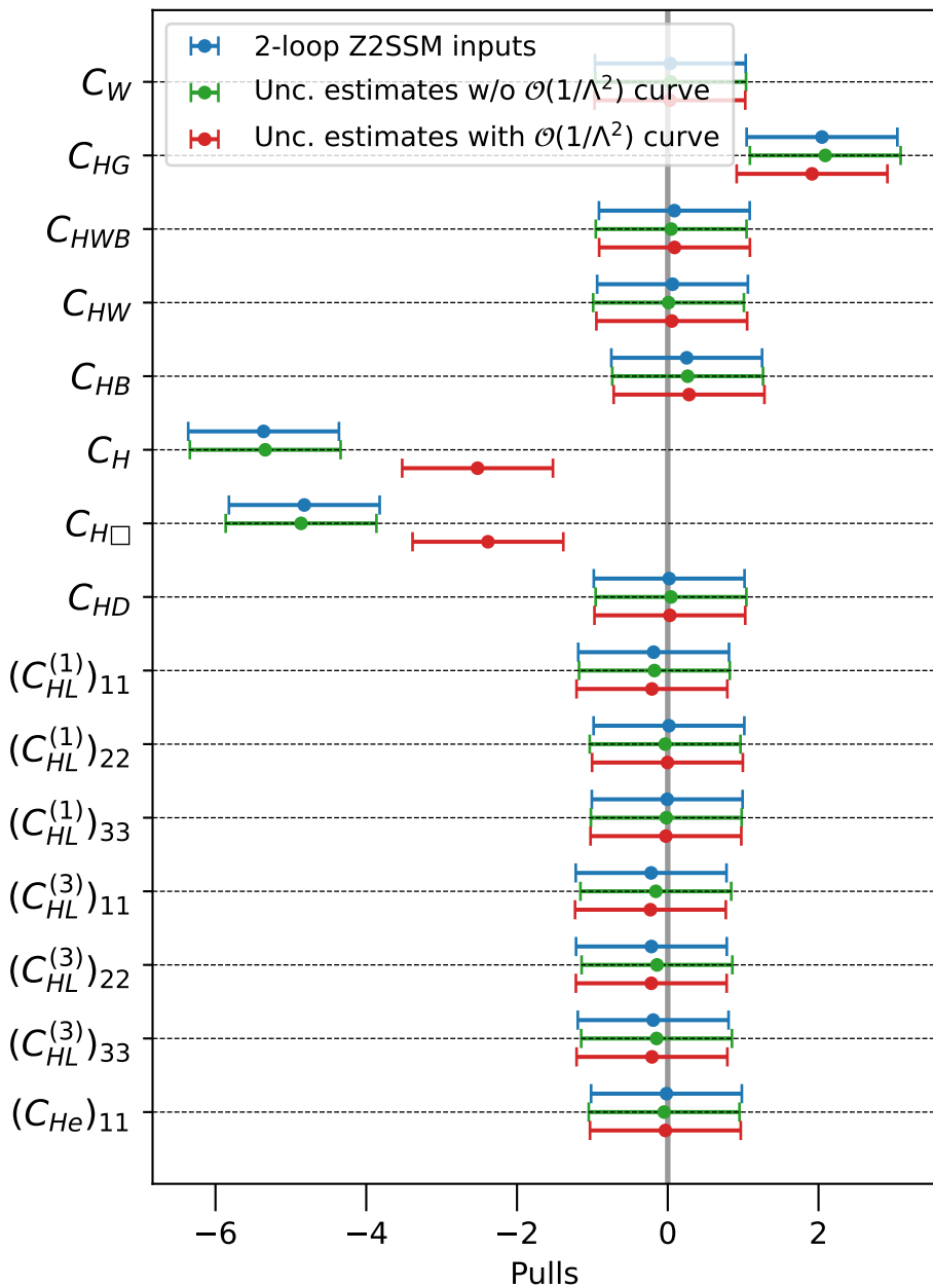
Z2SSM (BP 2), FCC-ee 240 + FCC-ee 365
