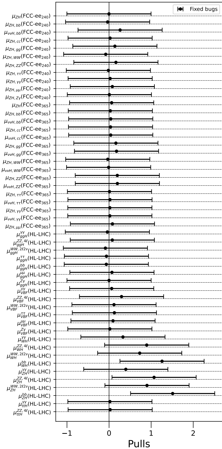
IDM (BP 1), FCC-ee 240 + FCC-ee 365
