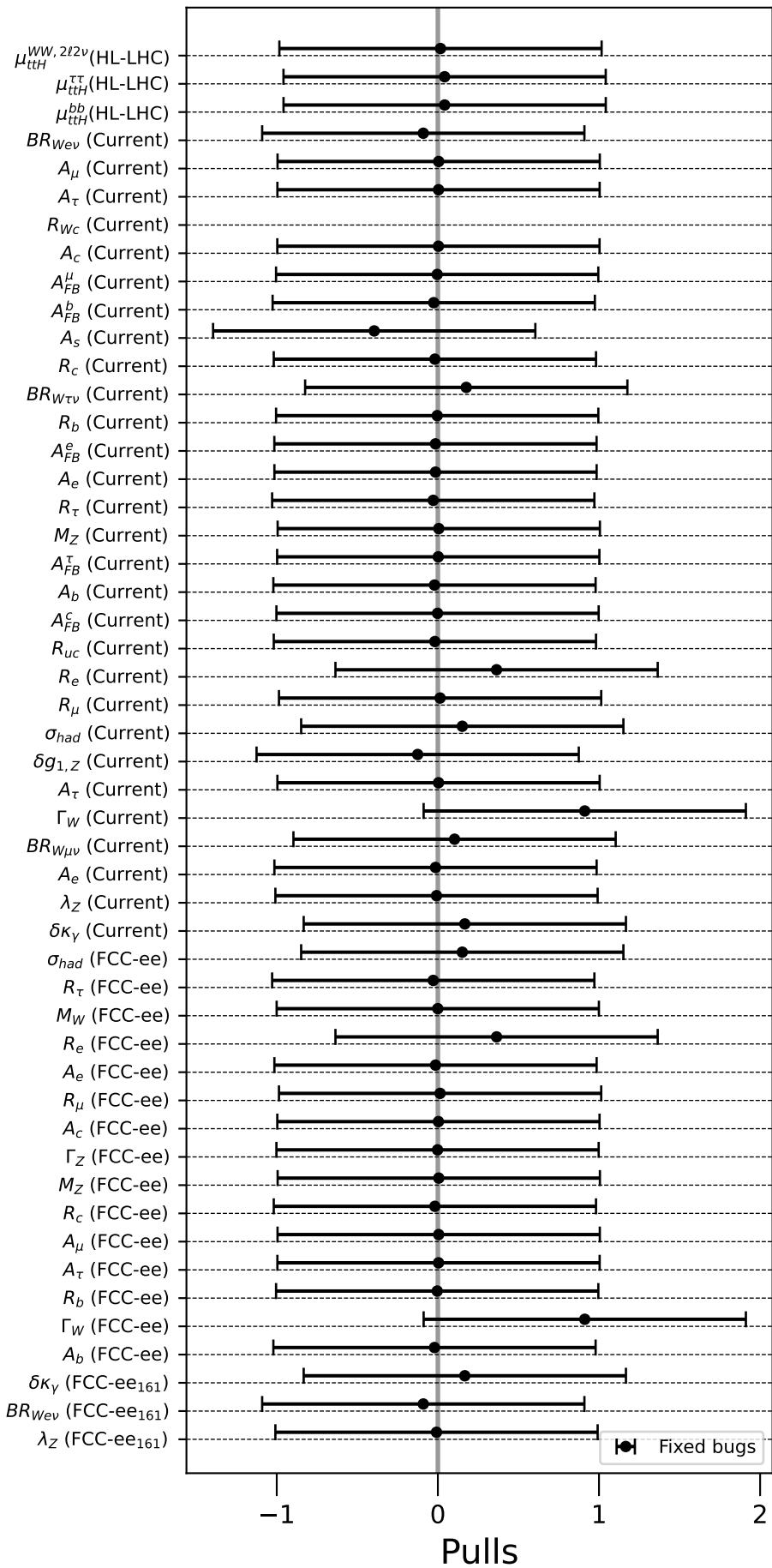
IDM (BP 3), FCC-ee 240 + FCC-ee 365
