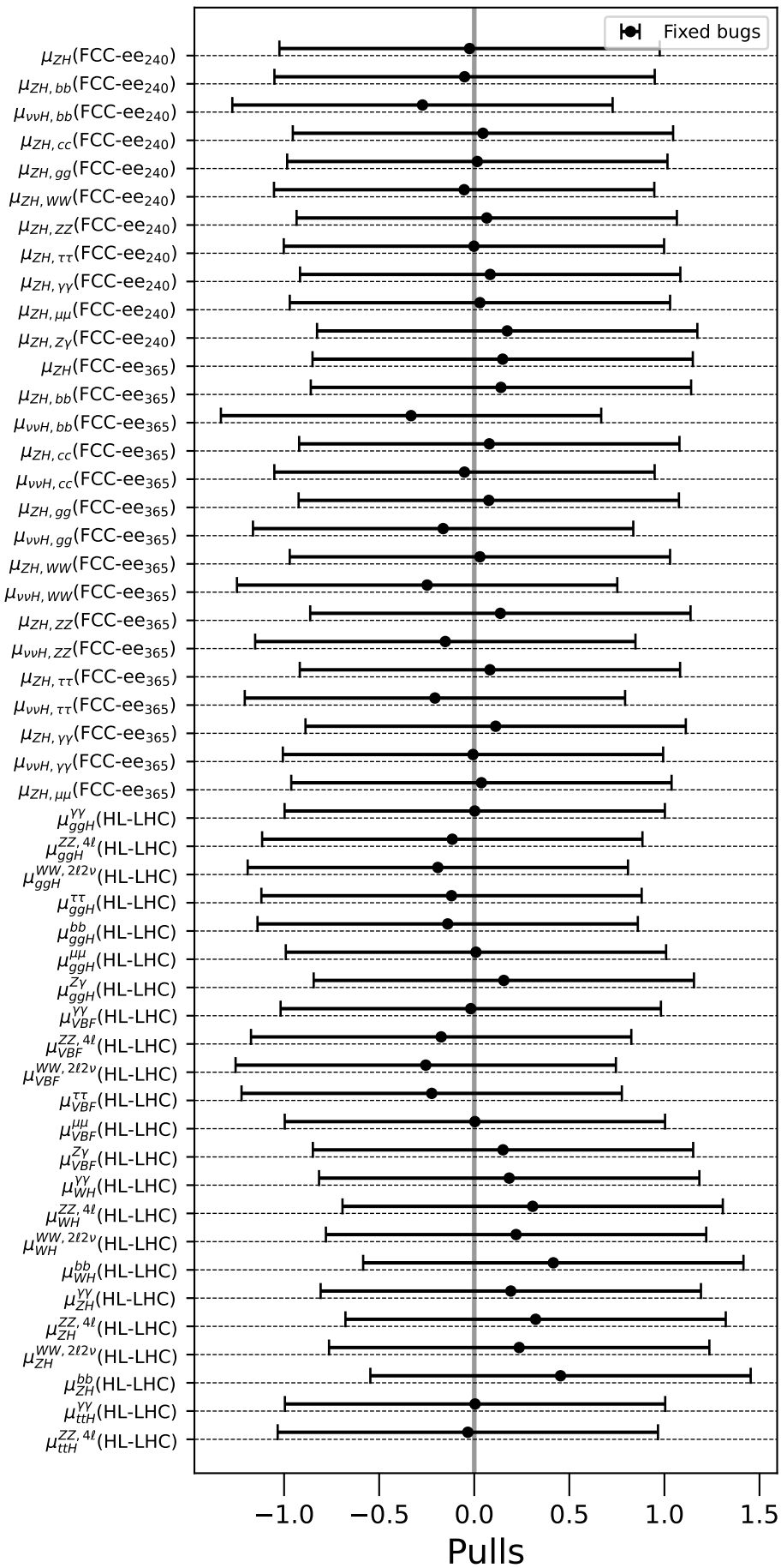
IDM (BP 0), FCC-ee 240 + FCC-ee 365
