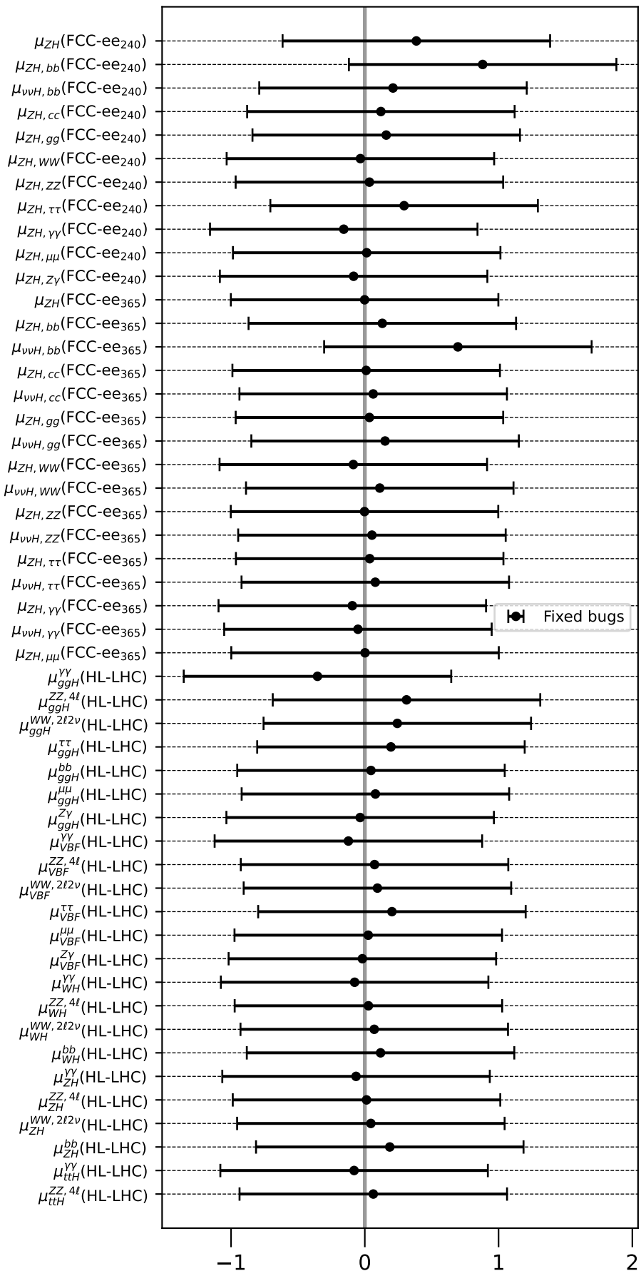
IDM (BP 1), FCC-ee 240 + FCC-ee 365
