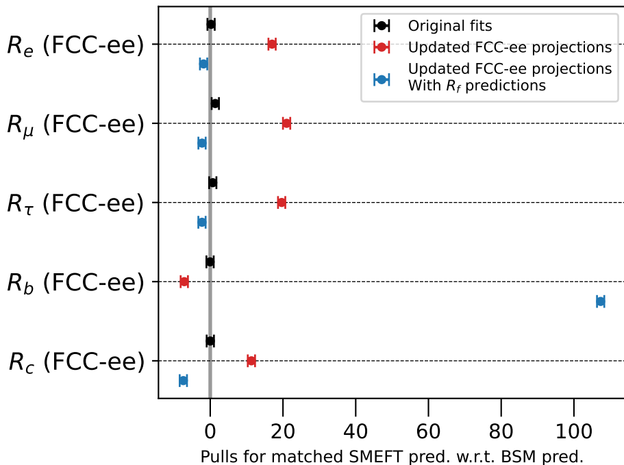
IDM (BP 3), FCC-ee 240 + FCC-ee 365
