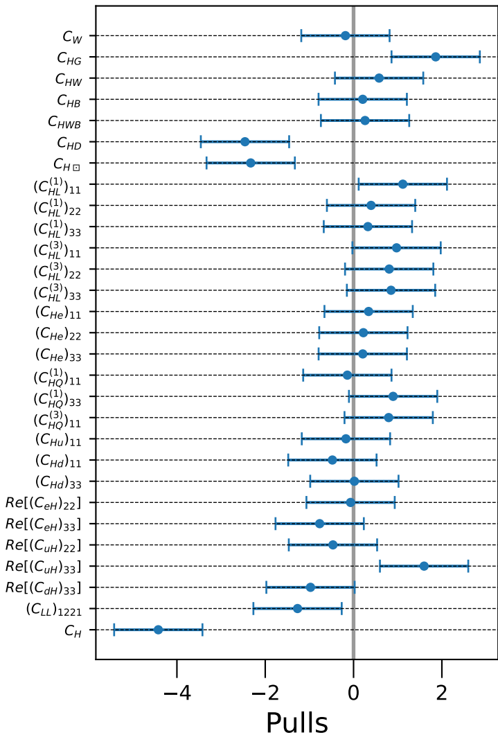
IDM (BPB 2), FCC-ee 240 + FCC-ee 365
