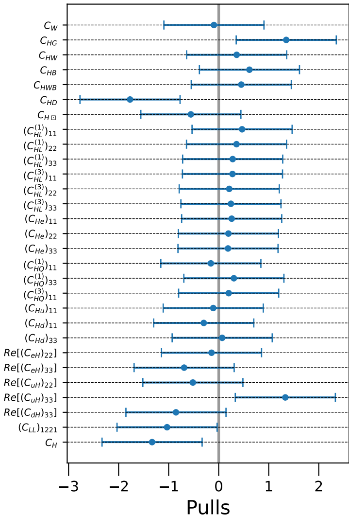
IDM (BP 1), FCC-ee 240
