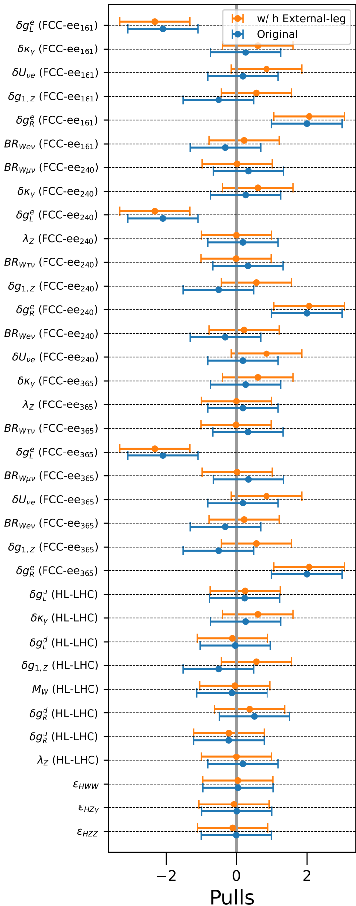
IDM (BP 1), FCC-ee 240 + FCC-ee 365
