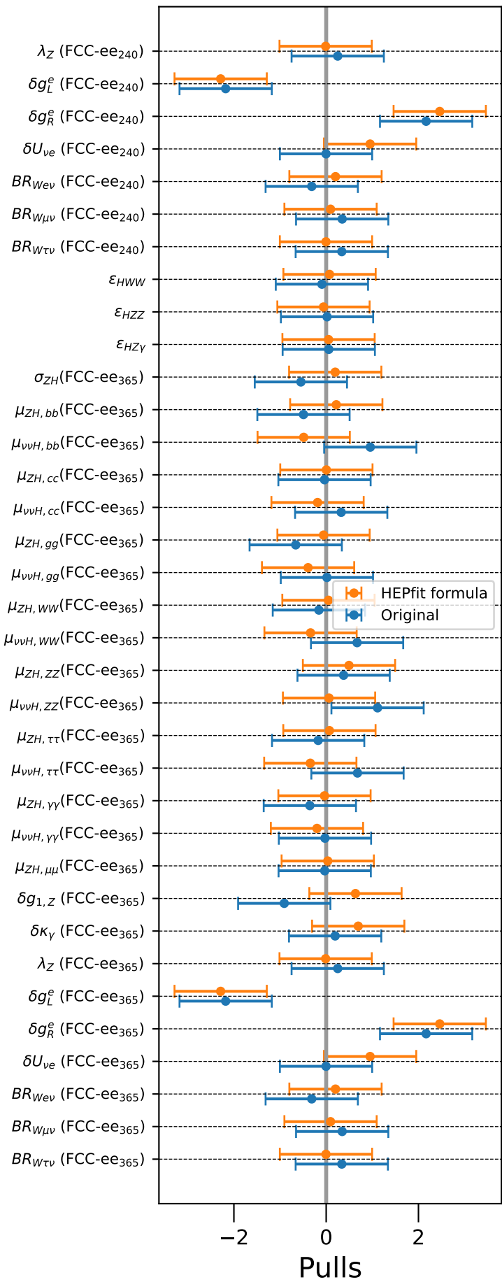
IDM (BP 2), FCC-ee 240 + FCC-ee 365
