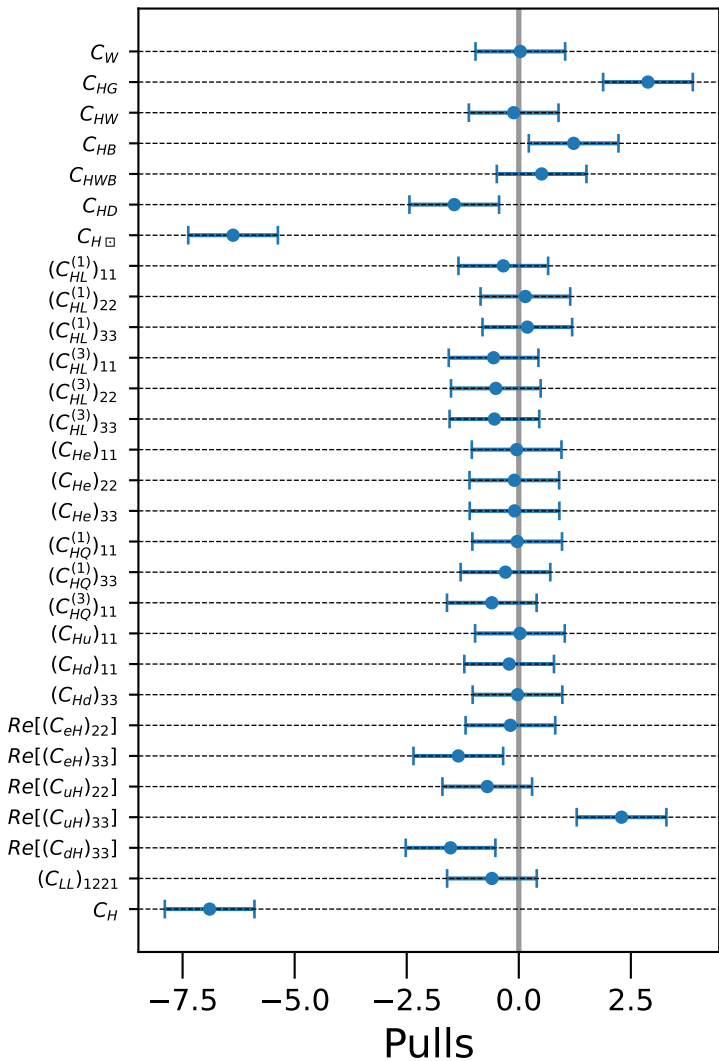
IDM (BP 3), FCC-ee 240 + FCC-ee 365
