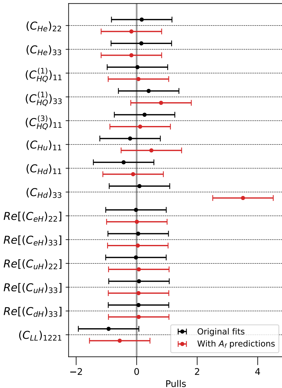
IDM (BP 0), FCC-ee 240 + FCC-ee 365
