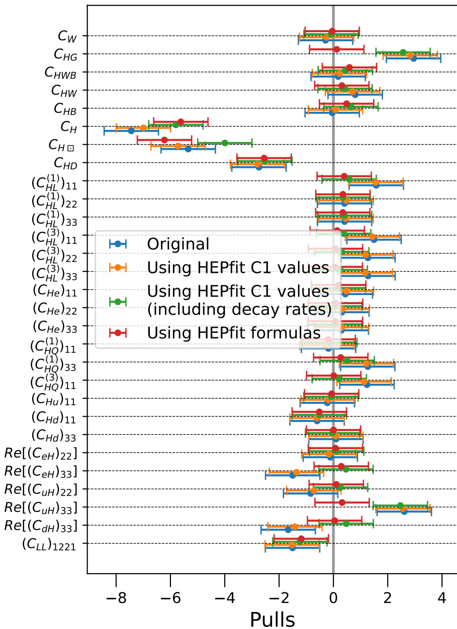
IDM (BP 2), FCC-ee 240 + FCC-ee 365
