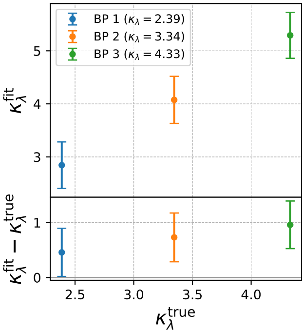
Using HEPfit C1 values
