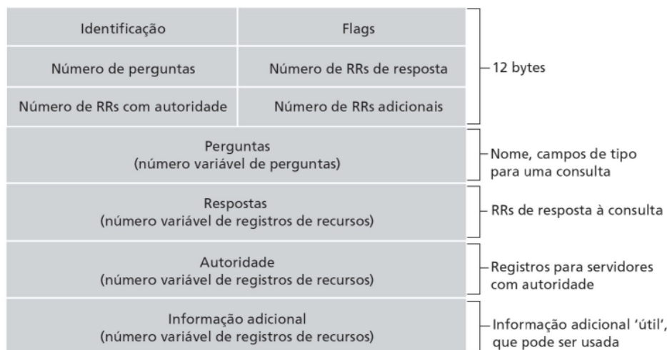
Figura 2.23 Formato da mensagem DNS
