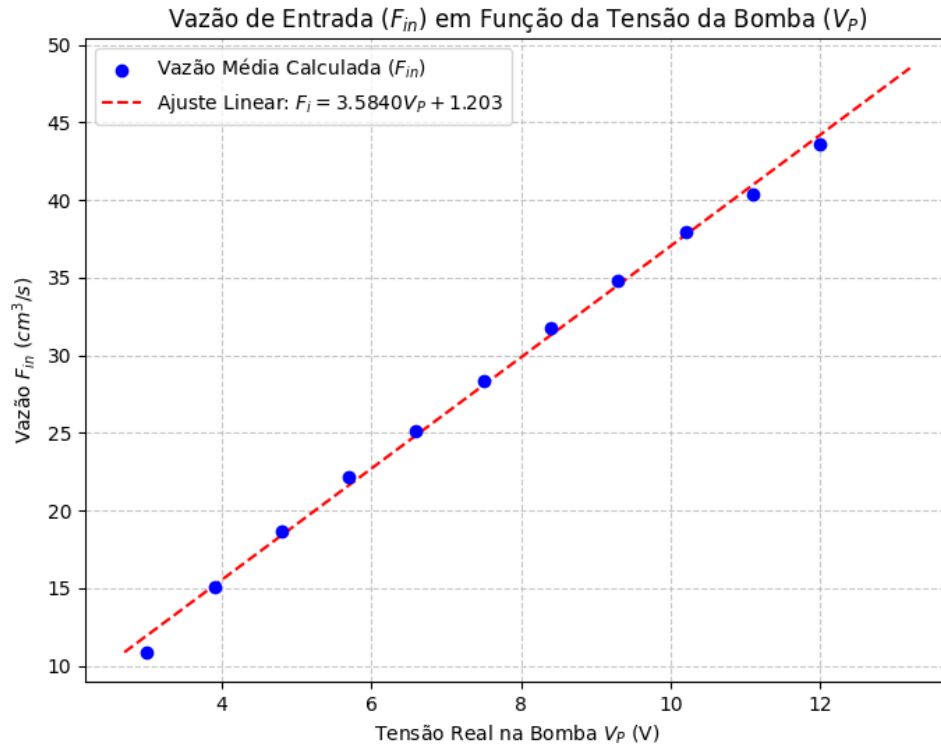
Figura 3: Curva da vazão de entrada com dispersão dos pontos e reta ajustada por mínimos quadrados.
