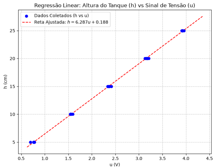
Figura 2: Curva estática do sensor de nível com dispersão dos pontos e reta ajustada por mínimos quadrados.
