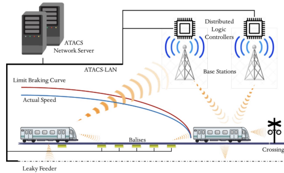
Abb. 1: Überblick über die Schieneninfrastruktur [Xia+20]
