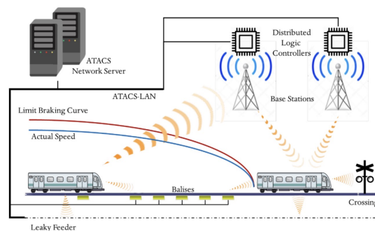
Abb. 1: Überblick über die Schieneninfrastruktur [Xia+20, S. 14]
