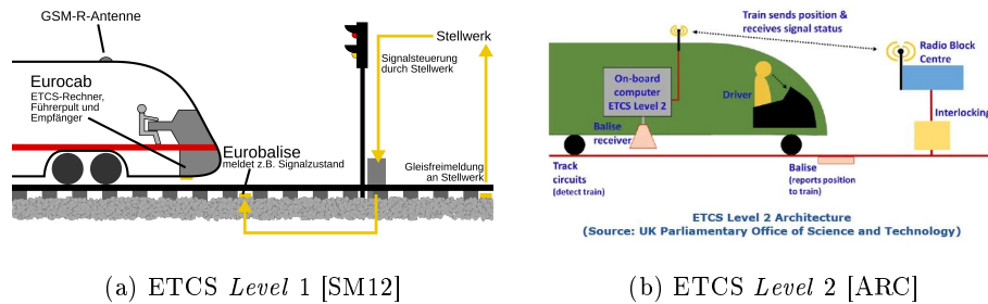
Abb. 2: ETCS Level 1 und Level 2
