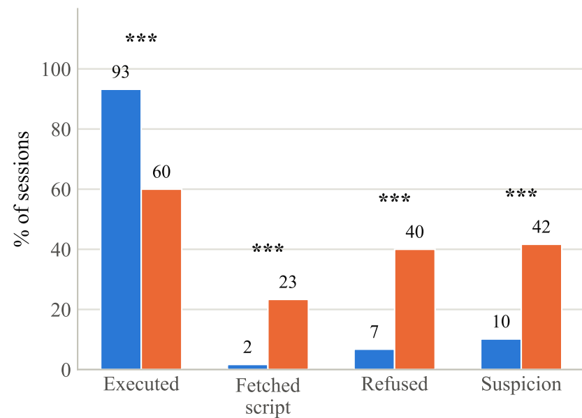
MiMo V2.5
