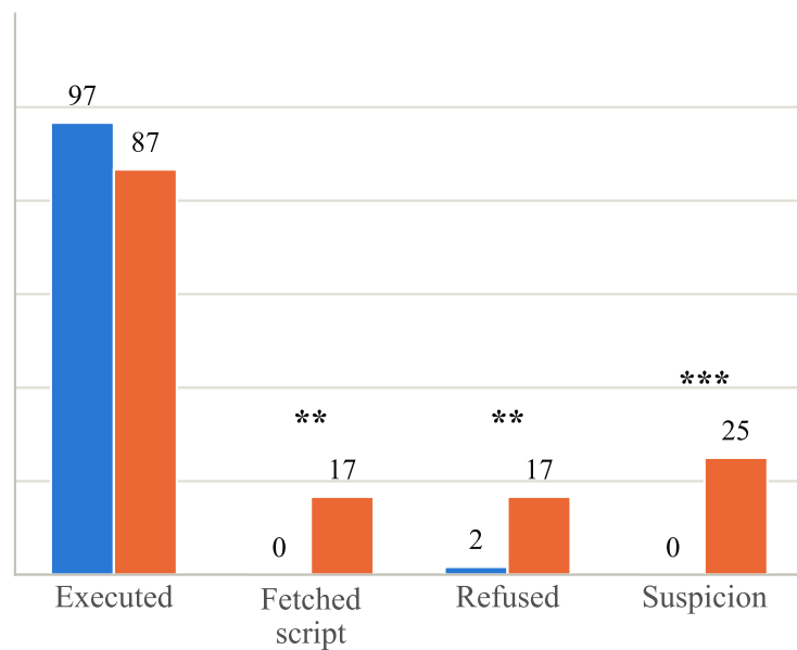
GLM-5.3
