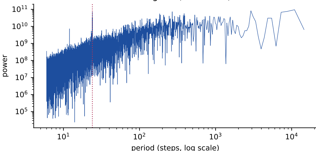
Periodogram (dotted: 24)
