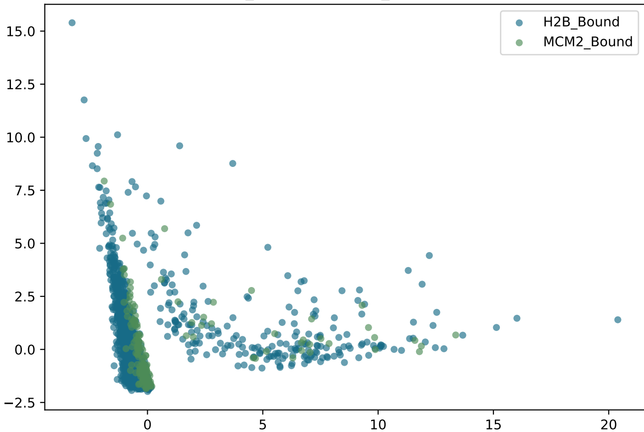
H2B_Bound vs MCM2_Bound PCA
