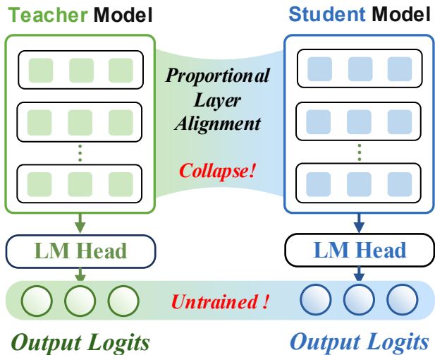
(b) Latent OPD
