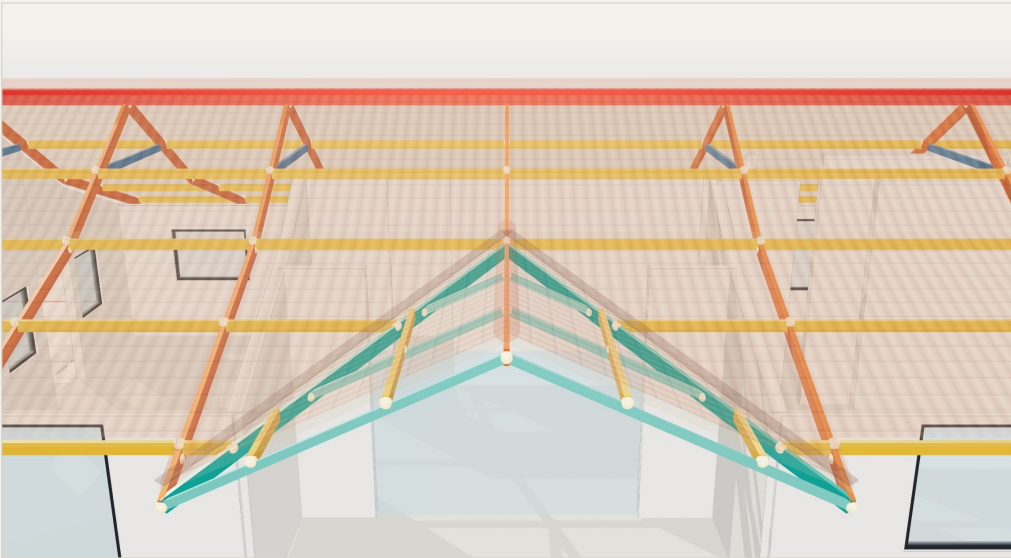
FRONTÓN – limahoyas y cerchuelas.
