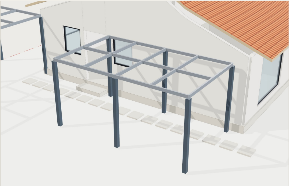
PÉRGOLA — 4,86 × 2,80 m. 4 vanos, eje central en 4 tramos.
