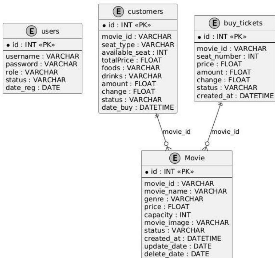
Hình 3. 7: ERD
