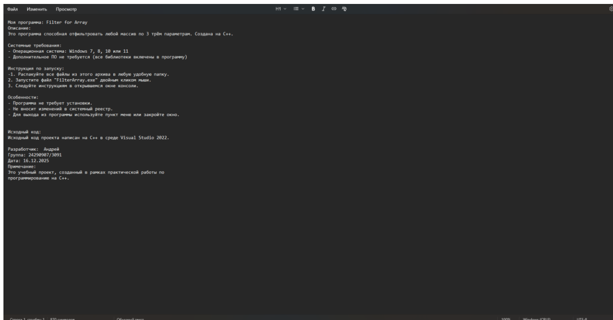
Рисунок 71 - Создание README-документа\
