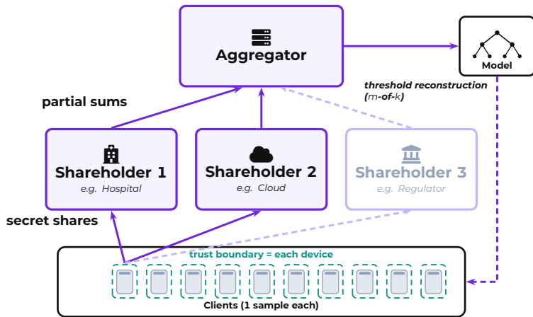
(b) PrivateBoost
